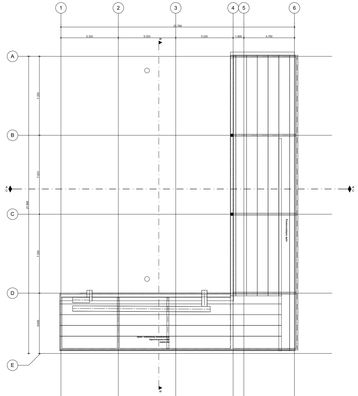
1. 1e verdieping 1:200
