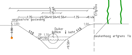
PROFIEL WATERGANG SCHAAL 1:50
