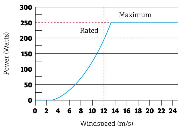
UWT - 0,75 M - 200 W
