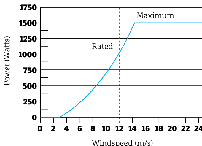
UWT - 1,5 M - 1000 W
