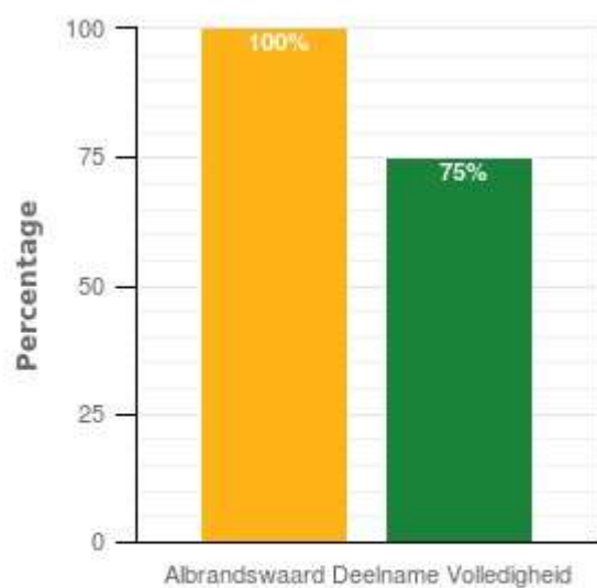
Deelscore Volledigheid
