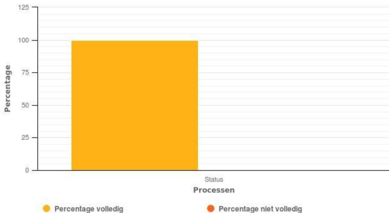
BAG 3.3 Volledigheid
