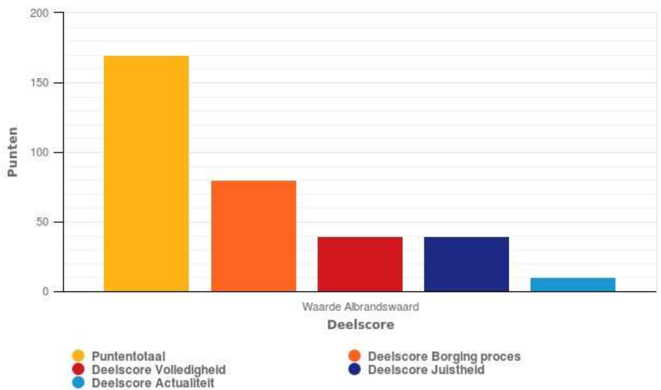
BAG 2.1 Overzichtsdiagram
